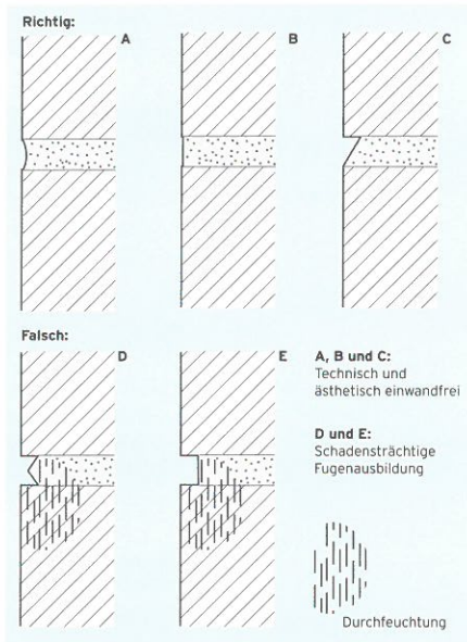
Bild 4: Günstige und ungünstige Verfüungsgeometrie
