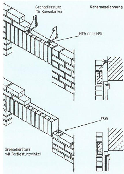
Bild 6: Grenadiersturzvarianten
