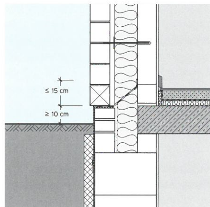
Bild 8: Fußpunktausbildung nach DIN 1996-2
