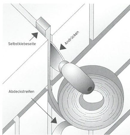
Bild 5: Dehnungsfuge mit imprägniertem Fugendichtungsband aus Schaumstoff
