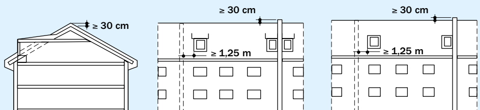
Bild 18 Brandwände im Dachbereich – Wohnungsbau (Länderunterschiede möglich), Auszug aus: Bayerische Versicherungskammer München, Brandwände und Öffnungen in Brandwänden, Anforderungen und Ausführung
