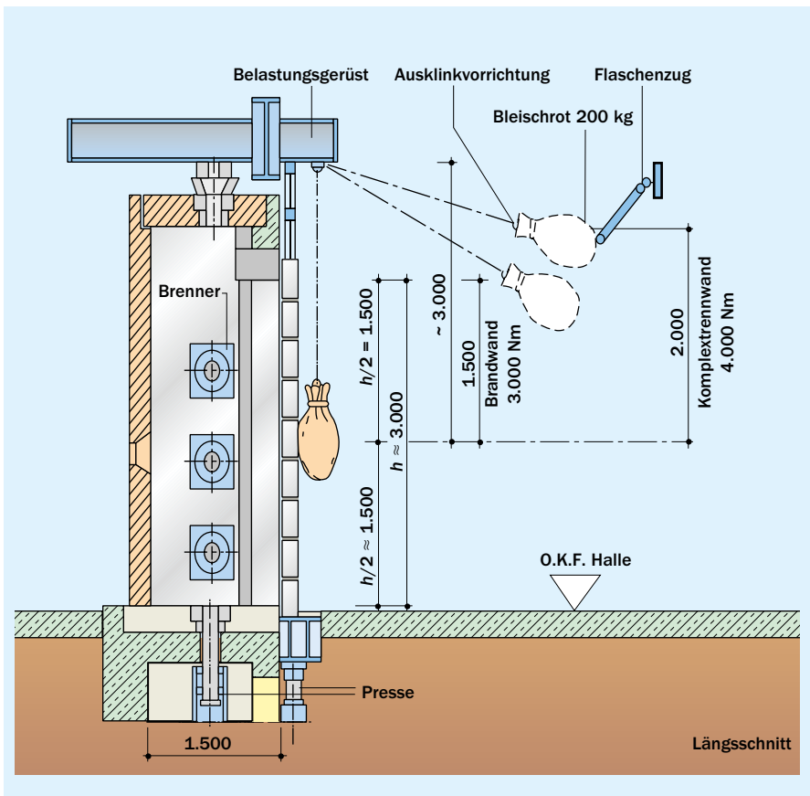
Bild 12 Prüfanordnung für Brandwände und Komplextrennwände nach den Prüfnormen
