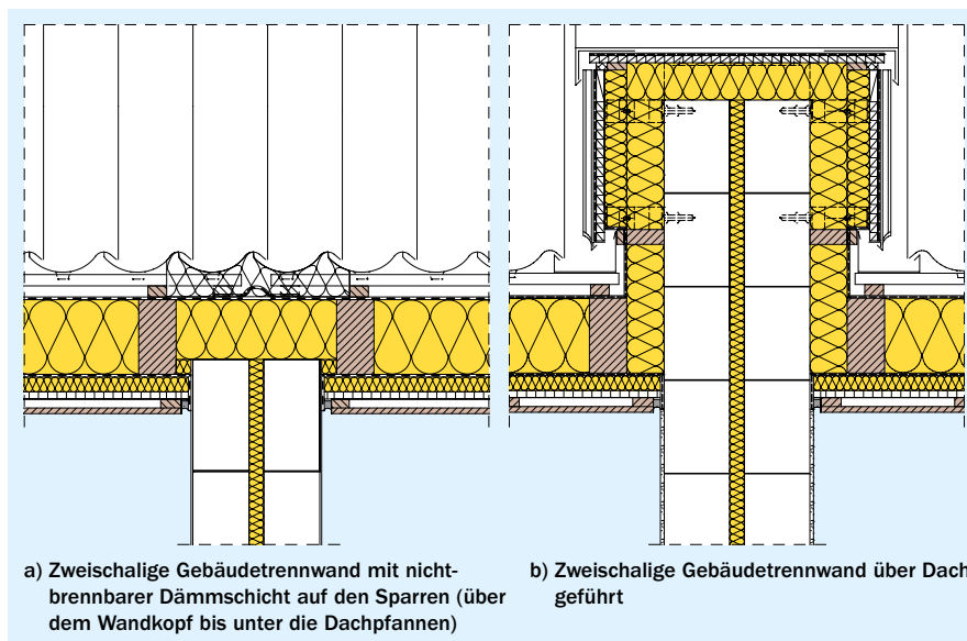
Bild 7 Gebäudeabschlusswand aus Kalksandstein-Mauerwerk im Dachbereich
