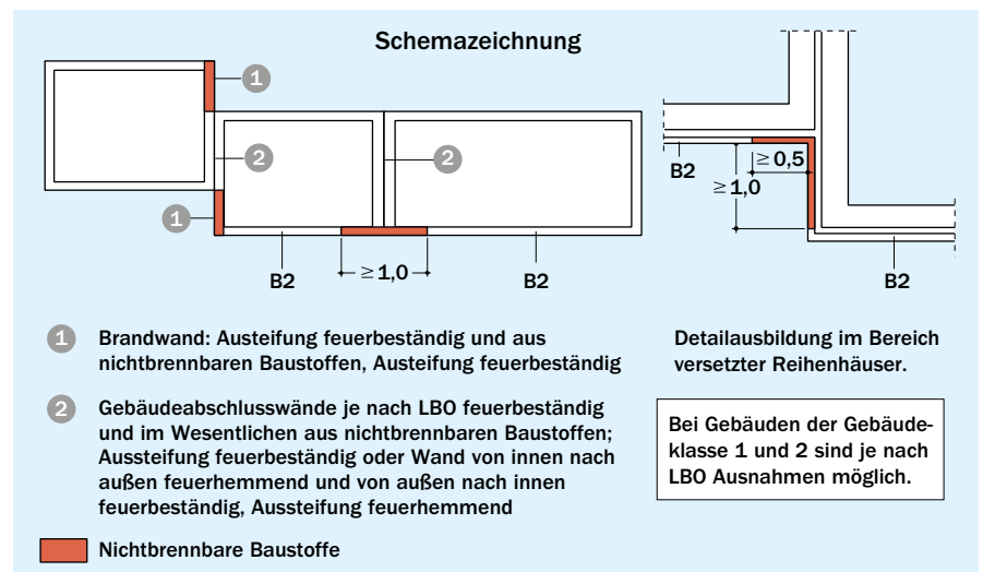
Bild 8 Beispiele für Regeln im Bereich der Gebäudetrennwände
