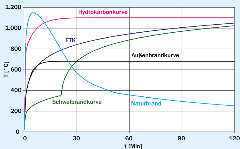
Bild 3 Temperaturprüfkurven – Brandeinwirkungen
