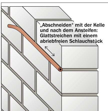
Bild 16: Fugenglattstrich
