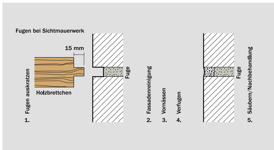
Bild 14: Nachträgliche Verfugung
