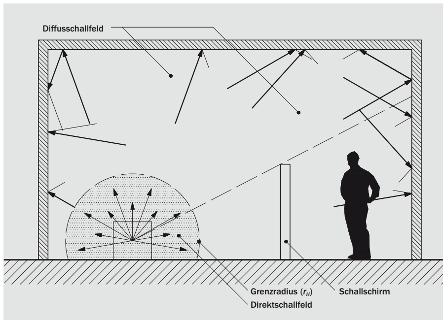
Bild 5: Diffuses Schallfeld
