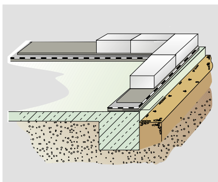
Bild 7/1: Anlegen der Kimmschicht
