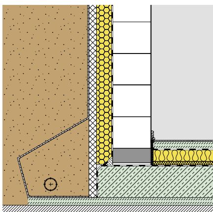
Bild 7/6: Detailsauflösung mit Wärmedämmung oberhalb der Bodenplatte
