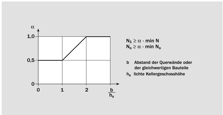
Bild 5/3: Abminderung des Mindestwertes der Wandlängskraft N_1 bzw. der Auflast N_0 bei zweiachsig gespannten Kelleraußenwänden
