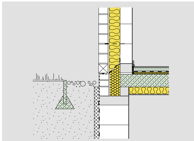
Bild 10/10: Unbeheizter Keller – Sockel-Anschluss, Kellerdecke außengedämmt, KS-Mauerwerk mit Kerndämmung und KS-ISO-Kimmstein
