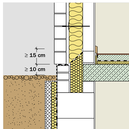
Bild 7/7: Sockelausbildung unterkellerten Häuser
