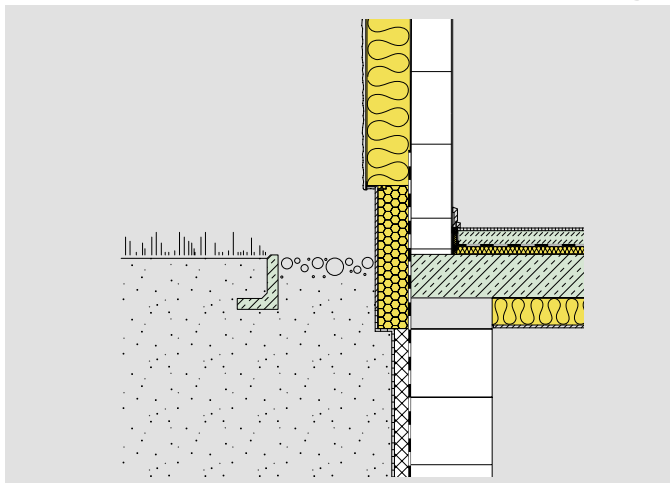
Bild 10/9: Unbeheizter Keller – Sockel-Anschluss, Kellerdecke außengedämmt, KS-Thermohaut mit KS-ISO-Kimmstein
