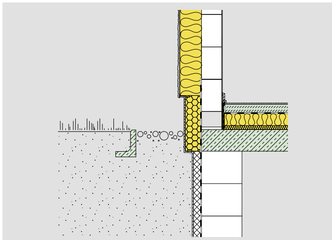
Bild 10/7: Unbeheizter Keller – Sockel-Anschluss, Kellerdecke innengedämmt, KS-Thermohaut mit KS-ISO-Kimmstein
