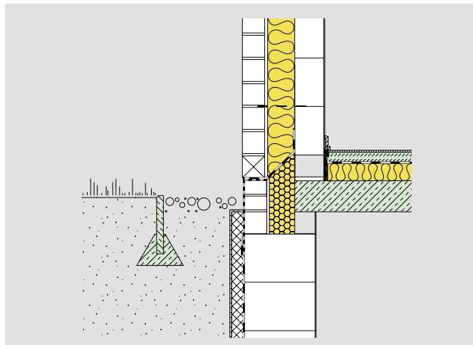
Bild 10/8: Unbeheizter Keller – Kellerdecke innengedämmt, KS-Mauerwerk mit Kerndämmung und KS-ISO-Kimmstein.
