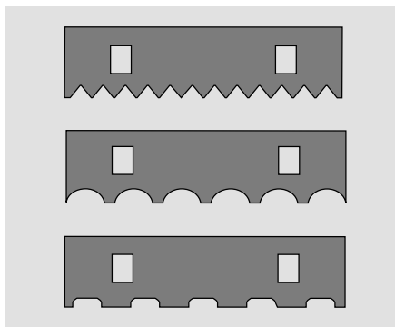
Bild 7/2: Beispiele verschiedener Zahnblechen für Dünnbettmörtel
