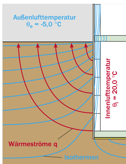
Bild 8/3: Wärmeübertragung über das Erdreich
