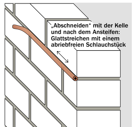
Bild 3/17: Fugenglattstrich
