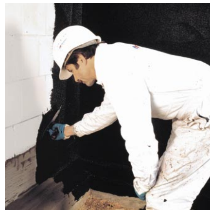
Bild 2/2: Die wasserdichte Abdichtung der Kelleraußenwand erfolgt durch qualifizierte Abdichtungsunternehmen.
