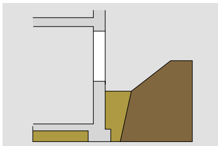
Bild 3/7: Kellerfenster an abgeboachter Geländeoberkante
