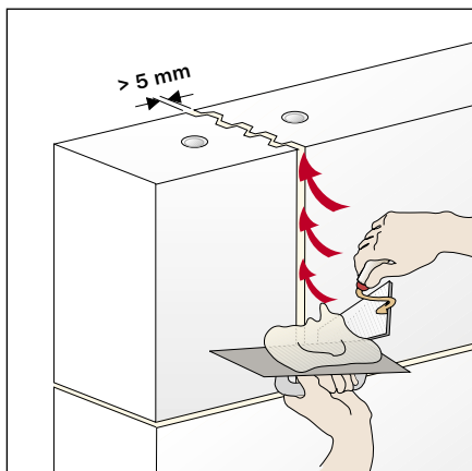
Bild 7/5: Vereinzelte auftretende Stoßfugen > 5 mm sind nach DIN 1053-1 zu schließen
