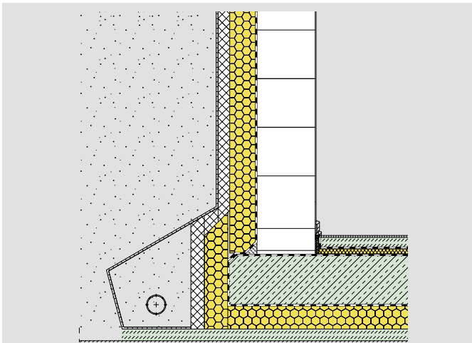
Bild 10/5: Beheizter Keller – Bodenplatte außengedämmt (Wärmedämmung nach Zulassung), KS-Kelleraußenwand außengedämmt
