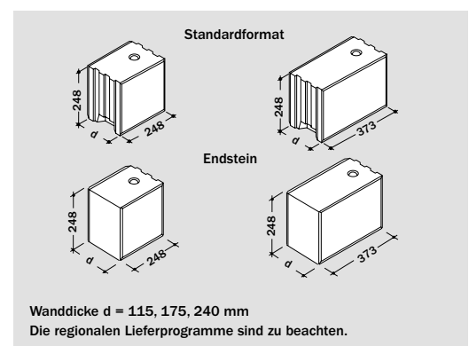
Bild 22: KS-Fasensteine
