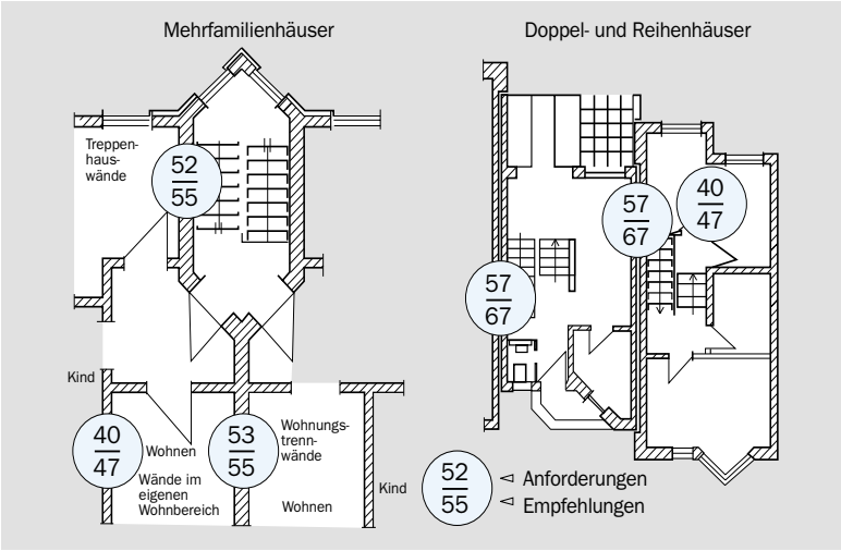
Bild 53: Anforderungen (obere Zahl) und Empfehlungen für den erhöhten Schallschutz (untere Zahl) an ausgewählten Grundrissen
