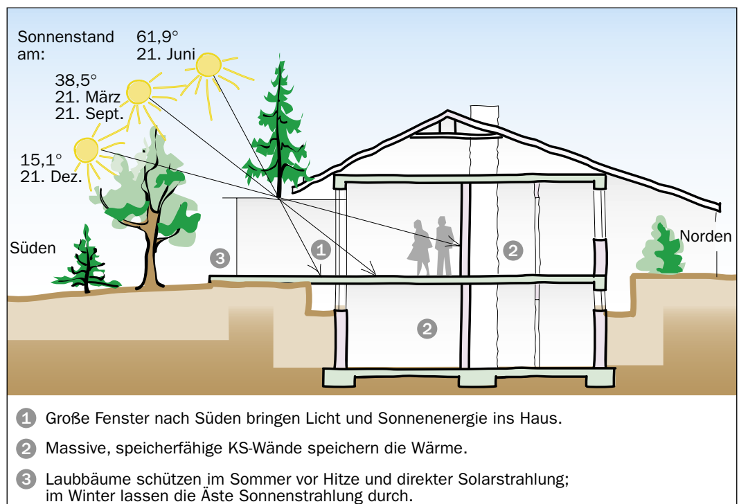
Bild 11: Nutzung der Sonnenenergie bei Energie sparendem Bauen [6]
