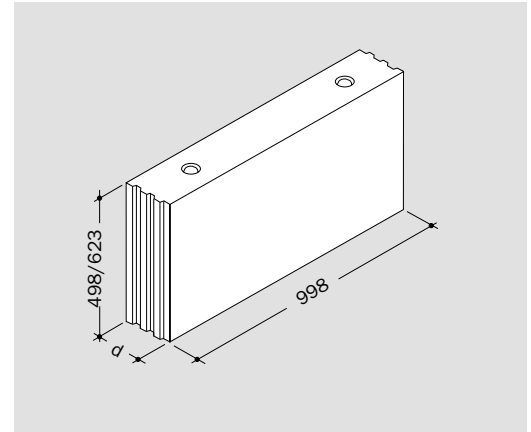
Bild 34: KS XL-Planelement
