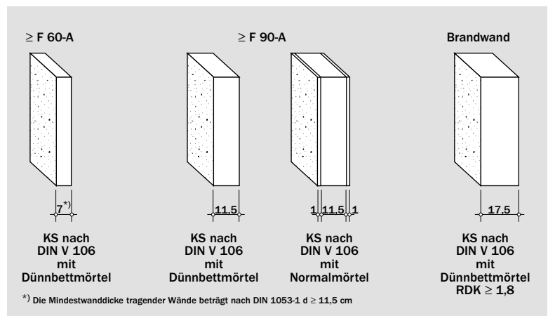
Bild 14: Kalksandstein-Konstruktionen weisen einen hohen Feuerwiderstand auf.
