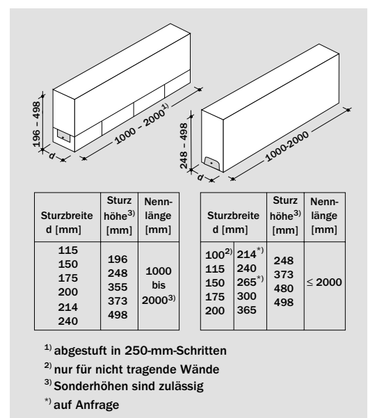
Bild 23: KS-Fertigteilstürze
