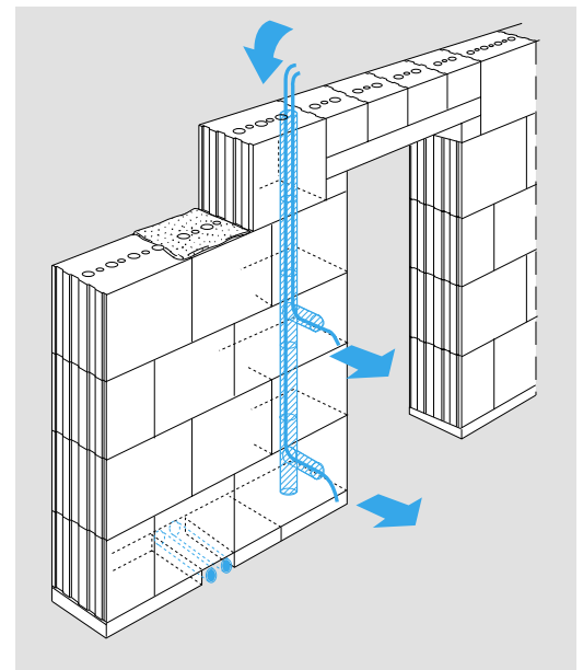
Bild 29: KS-Quadro E-Installationswand
