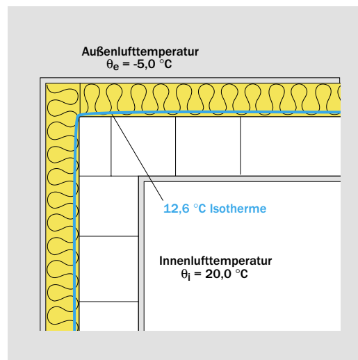
Bild 57: KS-Außenwände mit heute üblichen außen liegenden Wärmedämmstoffdicken von 12 cm lassen bei üblicher Nutzung (Raumlufthtemperatur 20^\circ \text{C} und 50 % relative Luftfeuchte) keine Schimmelpilzbildung zu.
