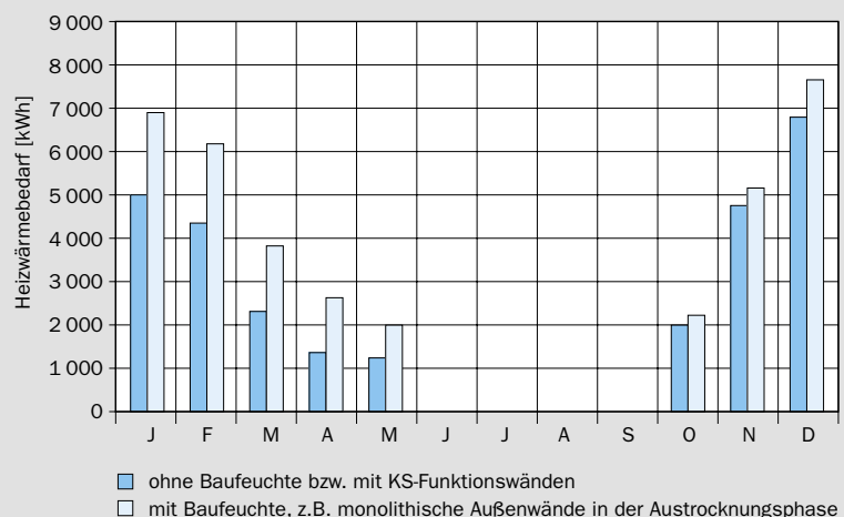
Bild 3: Heizwärmebedarf bei Gebäuden mit monolithischen Außenwänden mit bzw. ohne Baufeuchte. In der Austrocknungsphase (2 bis 3 Jahre) kann der Heizwärmebedarf um bis zu 30 % erhöht sein; nach [2].
