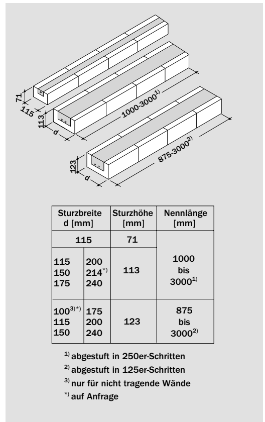
Bild 24: KS-Flachstürze
