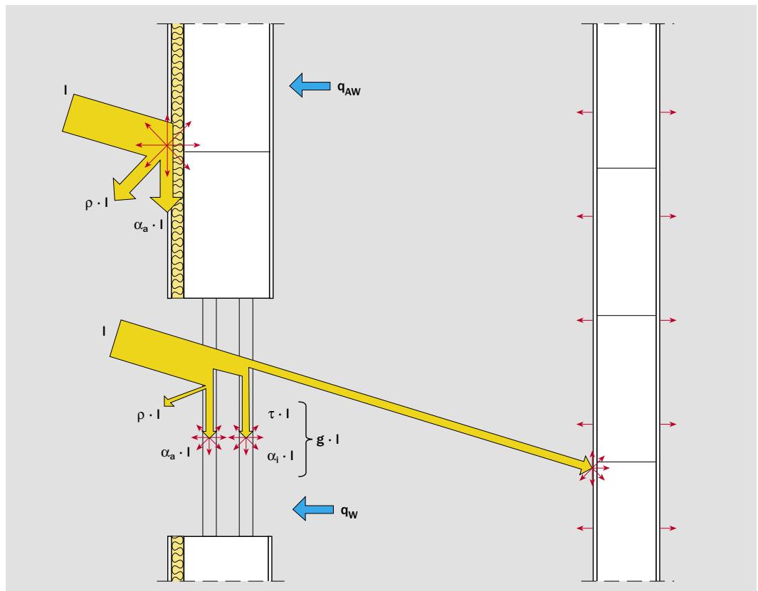
Bild 54: Hochwärmegeprägte KS-Außenwände vermindern Transmissionswärmeverluste im Winter. Massereiche KS-Wände innen und außen schützen im Sommer vor Überhitzung.
