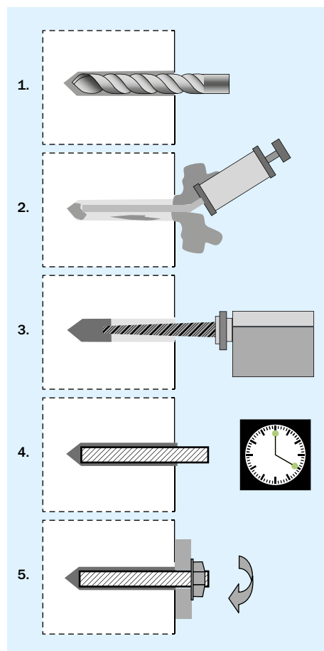
Bild 8 Montage eines Injektionsdübels als Vorsteckmontage
