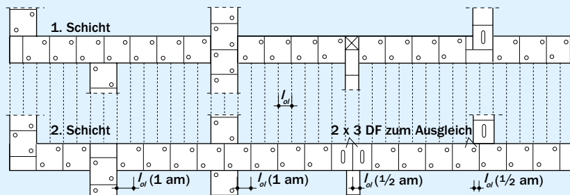
Bild 24 24 cm dicke Wand aus 4 DF(240) als Einsteinsmauerwerk
