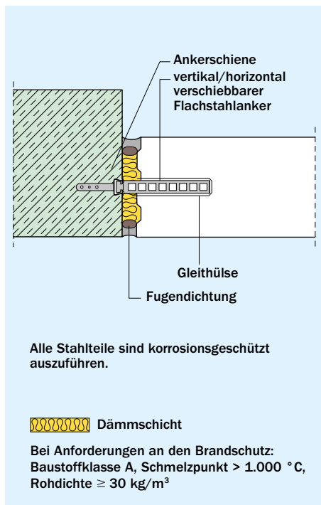
Bild 25 Beispiel für einen gelenkigen Wandanschluss an eine Stahlbetonstütze mit Ankerschienen mit Ankerschienenmörtel
