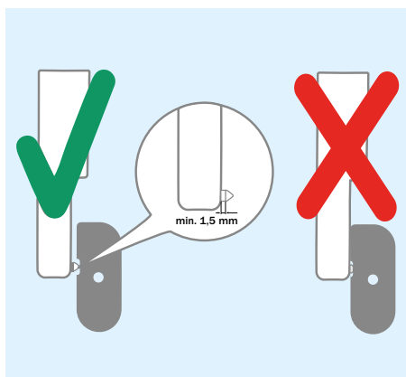
Bild 16 Korrektes Tragsystem der Versetzzange
