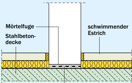
Vertikalschnitt
