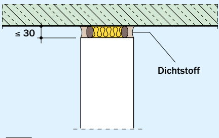
Schnitt
